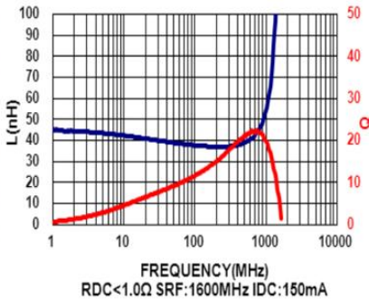
MHI0402D39NJT
