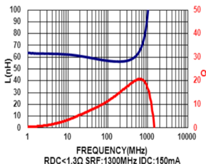
MHI0402D56NJT
