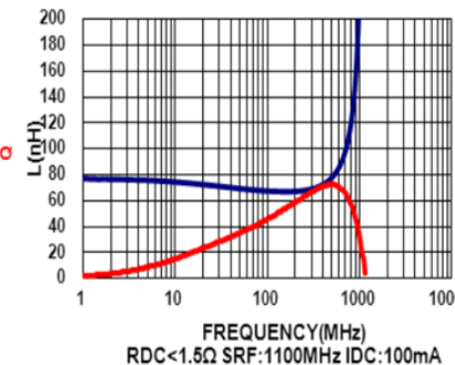
MHI0402D68NJT
